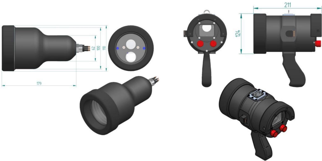
OceanSENSE ROV
