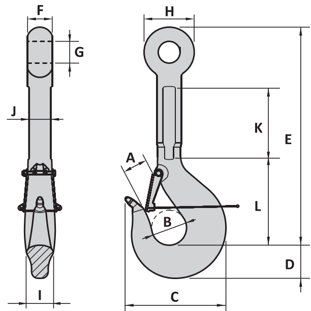
Type for Hook WLL 100 ton up to WLL 400 ton
