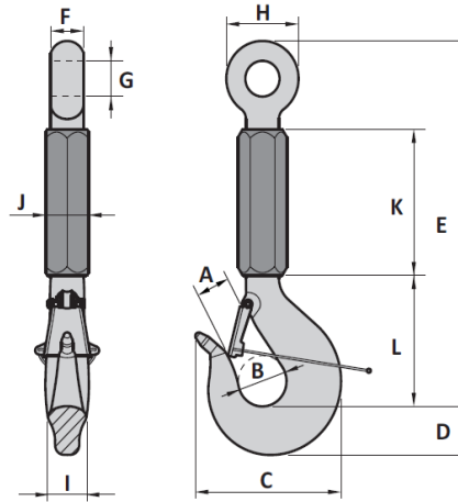
Type for Hook WLL 5 ton up to WLL 80 ton
